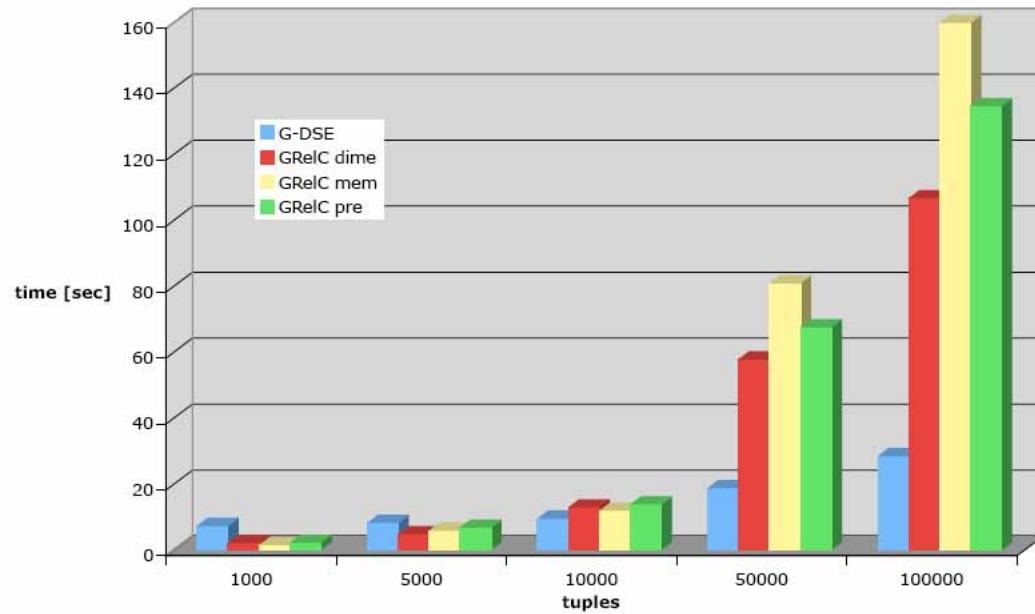
GDSE vs GRelC
